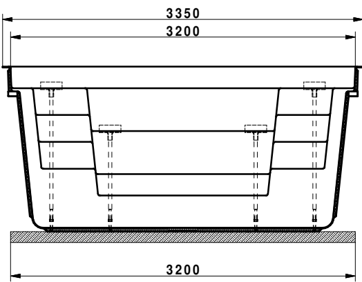
Schnitt B-B
