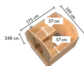
Fassauna asymmetrisch 1
