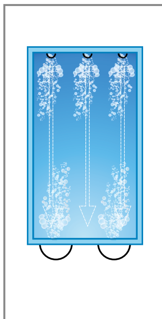
Längsdurchströmung mit 2 Einbau-Skimmern und 3 Einlaufdüsen
